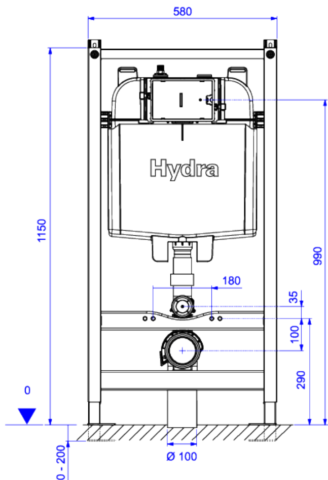
Desenho Técnico
