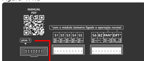
Figura 4.4.b Indicador do Pino 1
