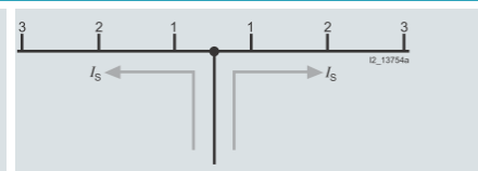
Alimentação ao longo do barramento ou ponto médio de alimentação: A soma da corrente de saída por ramo (1, 2, 3 ... n) não deve ser maior do que a corrente máxima por fase, IS/fase.
