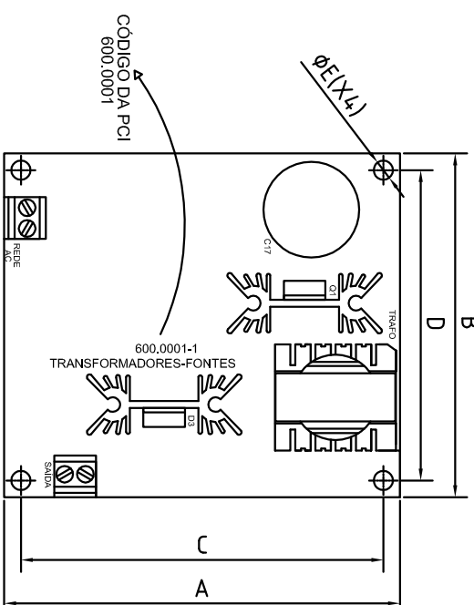
Vista Superior
