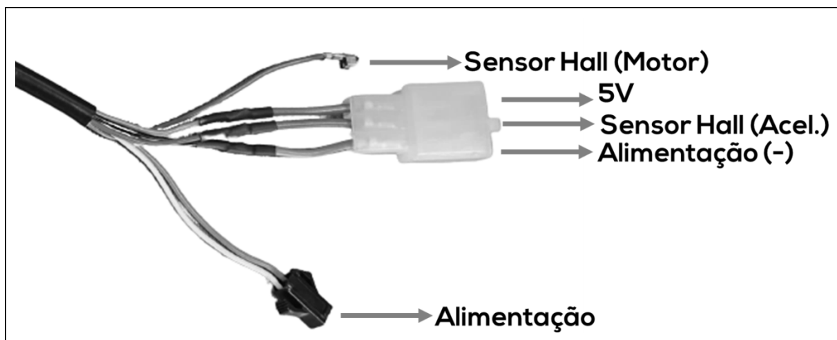
Figura 2 – Diagrama Elétrico do display LCD9.
