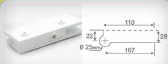
Dobradiça superior
