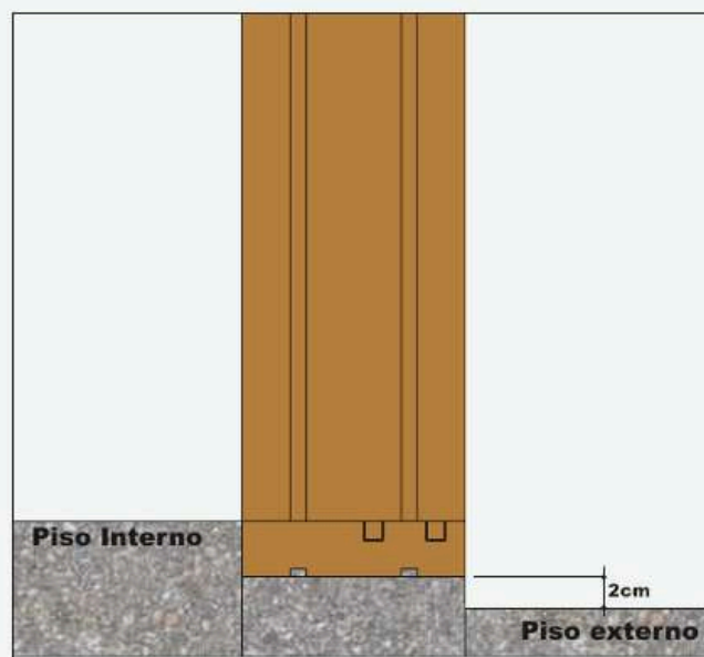
FIGURA 9 - VÃOS DE PORTAS EXTERNAS DEVEM ESTAR 2CM ACIMA DO PISO EXTERNO.
