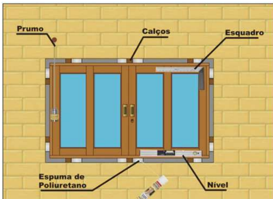
FIGURA 2 - INSTALAÇÃO DA ESQUADRIAS
