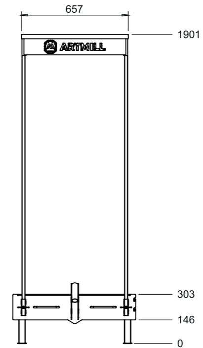
VISTA LATERAL
