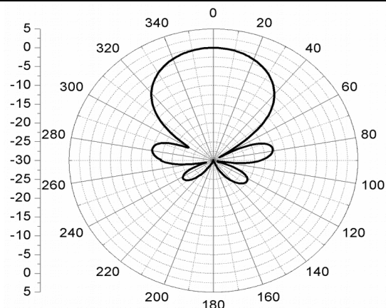
Diagrama de Radiação @380 MHz Plano - E Radiation Pattern @380 MHz – E Plane
