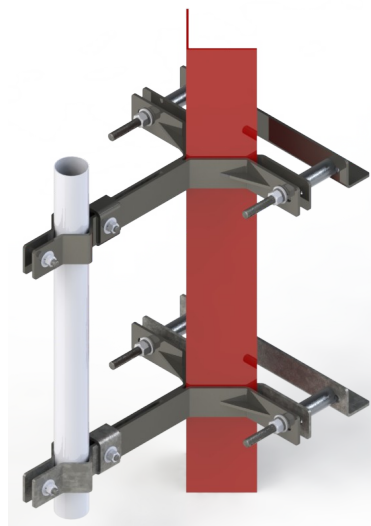
Fixação Cantoneira 4"
