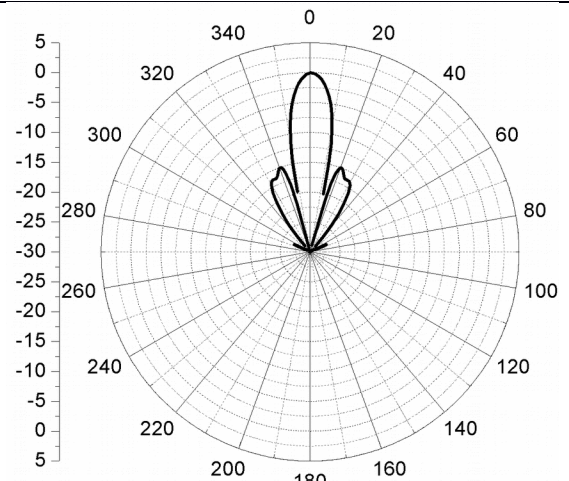
Diagrama de Radiação @925 MHz Plano - E Radiation Pattern @925 MHz – E Plane
