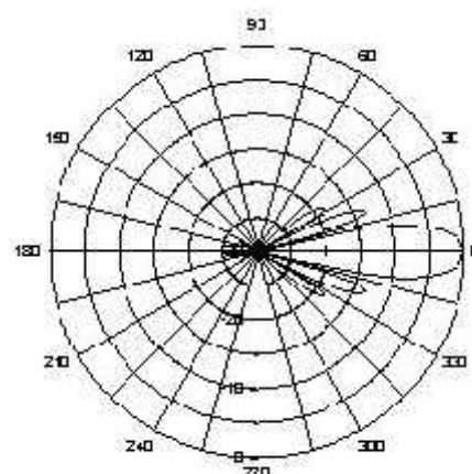
Diagrama de Radiação @433 MHz Plano - E Radiation Pattern @433 MHz – E Plane
