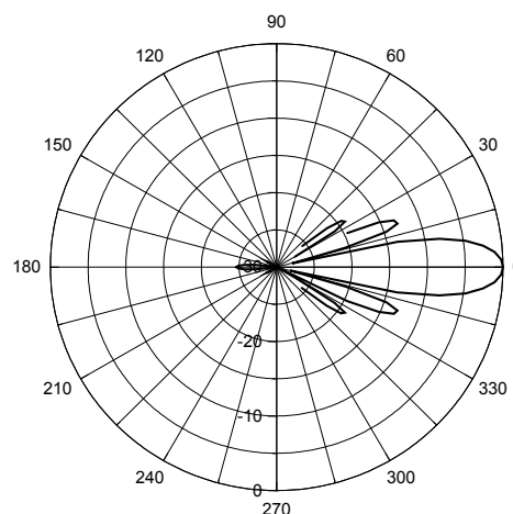
Diagrama de Radiação @380 MHz Plano – H
