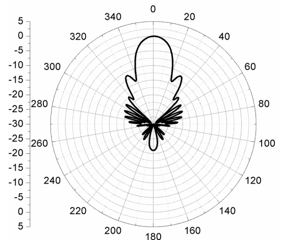
Diagrama de Radiação @830 MHz Plano - E Radiation Pattern @830 MHz – E Plane
