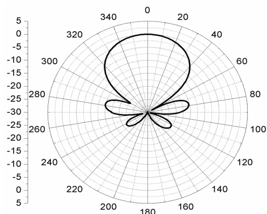
Diagrama de Radiação @380 MHz Plano - E Radiation Pattern @380 MHz – E Plane
