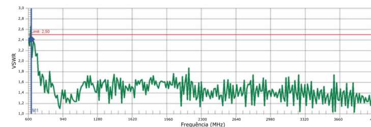
EXEMPLO: Gráfico de VSWR de uma Antena AP8900
